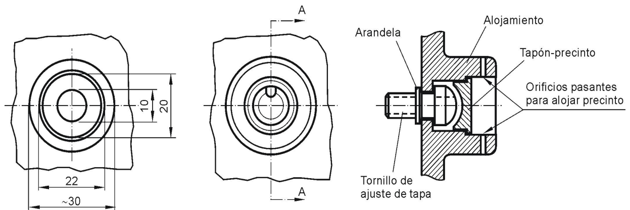
Figura 2 - Alojamiento para tapón-precinto del tornillo.
