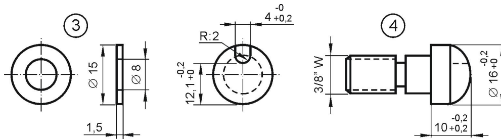
Figura 1 - Tornillo de ajuste de la tapa (con cabeza especial).
