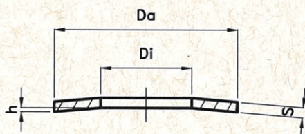
ARANDELA CONICA ELASTICA
